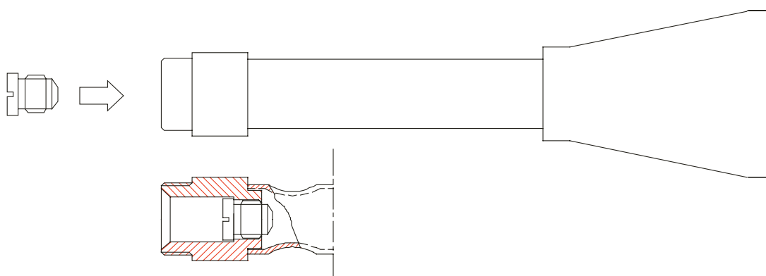
Rys. 9.4 Położenie dyszy
