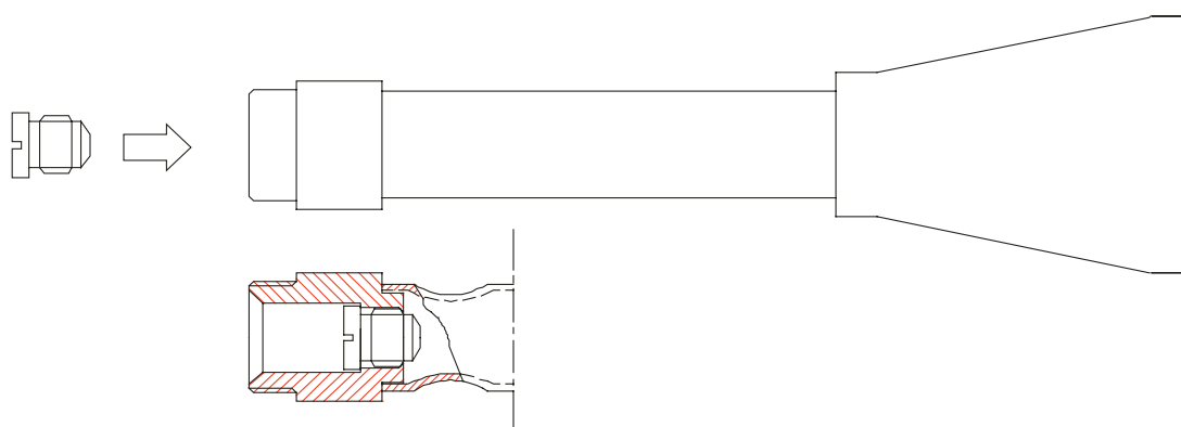
Rys. 9.4 Położenie dyszy
