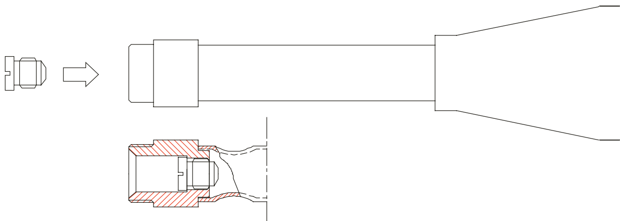
Rys. 3.8 Położenie dyszy
