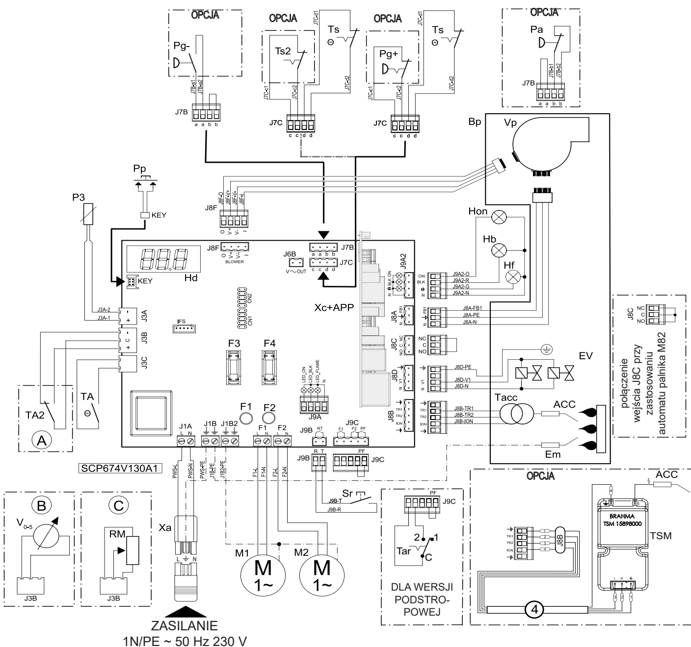
Rys. 3.2 Wyposażenie elektryczne
