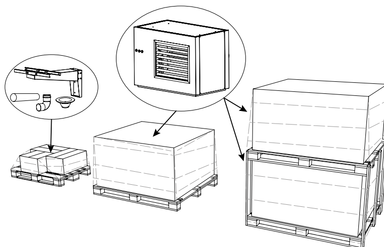
Rys. 1.1 Pakowanie urządzeń
