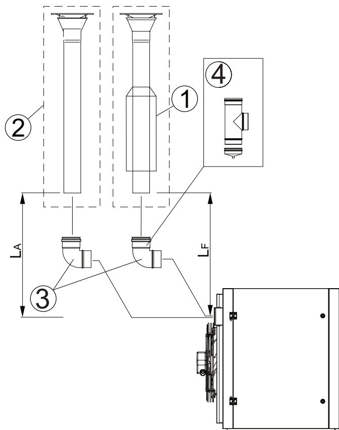
Rys. 6.5 System spalino-powietrzny typ C33 pionowy
