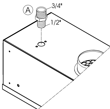
Rys.7.1 Podłączenie do gazociągu za pomocą przyłącza elastycznego 1/2" lub 3/4" (minimalna długość 50 cm)
