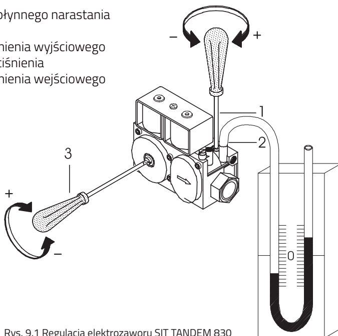
Rys. 9.1 Regulacja elektrozaworu SIT TANDEM 830
