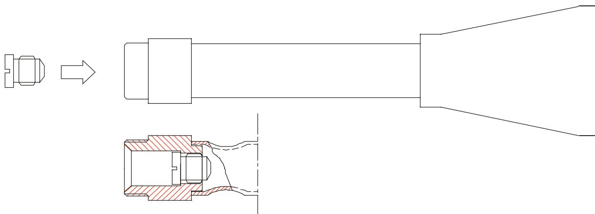
Rys. 3.8 Położenie dyszy
