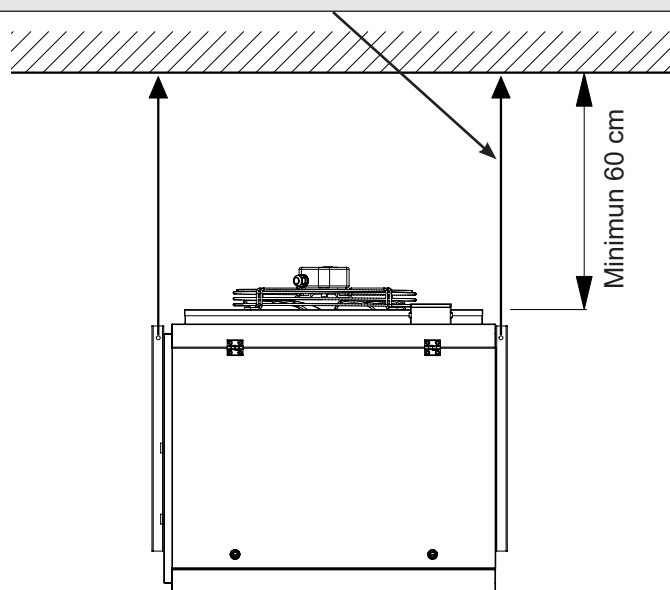
Rys. 5.13 Zawieszenie sufitowe
