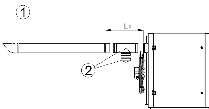
Rys. 6.4 Przewody spalinowe B23 ściennie (Eolo 85 / 100)
