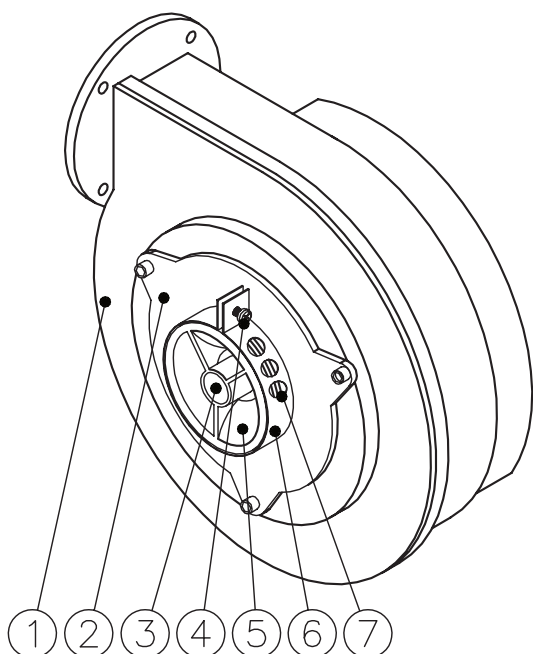
Rys. 7.3 Dmuchawa gazowa palnika
