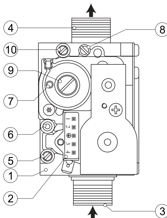
Rys. 7.1 Elektrozwór 848 Sigma
