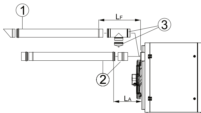
Rys. 6.2 System spalino-powietrzny typ C13 ścienny (Eolo 85 e 100)
