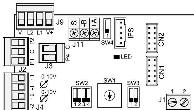
Rys. 3.15 Płyta komunikacyjna slave SCP674V202
