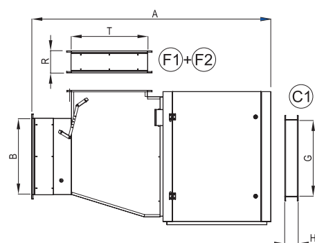
Widok boczny
