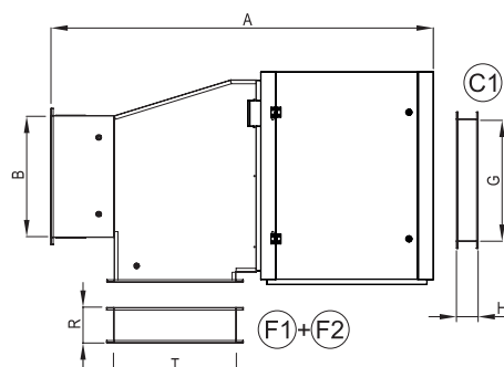
Widok boczny
