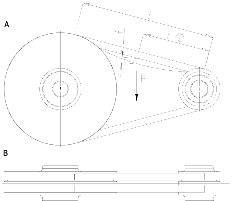
Rys.7.2. Oznaczenia wymiarów do wykresu siły naciągu pasów.
